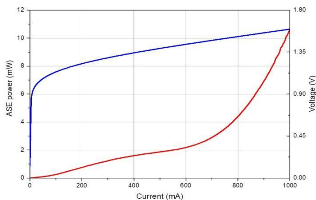
L-I-V 曲线
