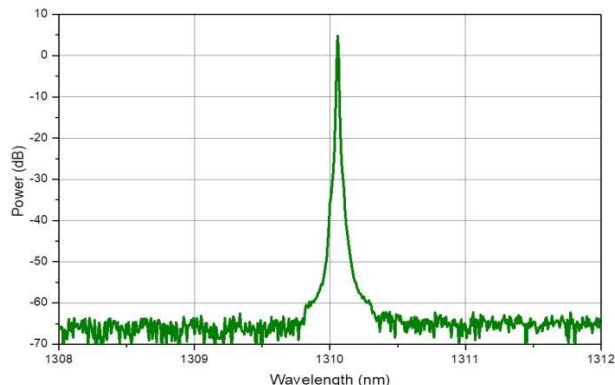
光谱(res. 10pm)
