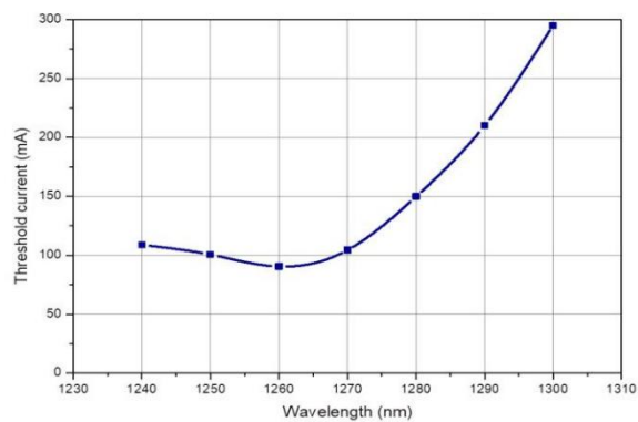
阈值电流
